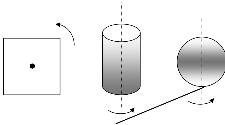
Συμμετρία περιστροφής
